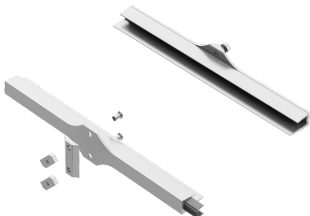
A set for 8 mm (0,31") glass shelf / Ein Set für 8 mm (0,31") Glas L = 320 mm nr 038 017 05
